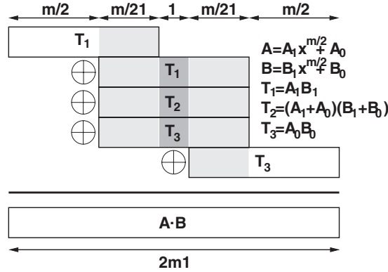
Fig. 4. Karatsuba multiplication
