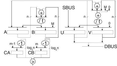
Fig. 8. Divider.
